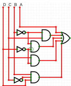
Gambar 3.5 Rangkaian logika fungsi (12) (Sumber: Arsip pengguna)
