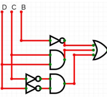
Gambar 3.3 Rangkaian logika fungsi (10) (Sumber: Arsip pengguna)
