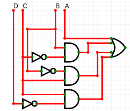
Gambar 3.8 Rangkaian logika fungsi (15) (Sumber: Arsip pengguna)
