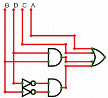
Gambar 3.2 Rangkaian logika fungsi (9) (Sumber: Arsip pengguna)
