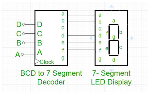
Gambar 2.4 Ilustrasi proses dari dekoder ke seven segment display
