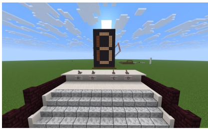
Gambar 5.2 Tampilan input = 3 atau 0011 (Sumber: Arsip pengguna)
