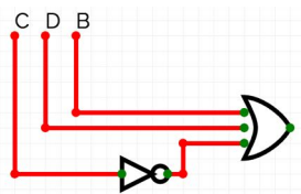
Gambar 3.4 Rangkaian logika fungsi (11) (Sumber: Arsip pengguna)
