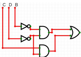
Gambar 3.6 Rangkaian logika fungsi (13)
