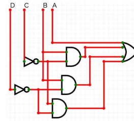
Gambar 3.7 Rangkaian logika fungsi (14) (Sumber: Arsip pengguna)
